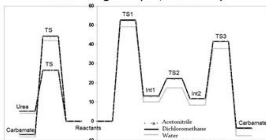
Perfil energético ( \Delta G , kcal mol -1 )
